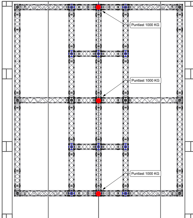
3-Puntsbelasting
